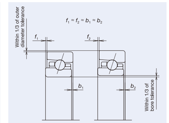
Fig. 3.11 DU Combination
