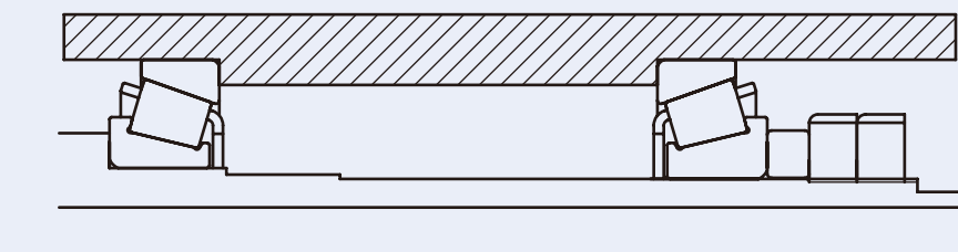
(d) Position preload without spacers
