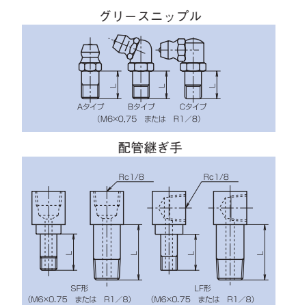
図 3 給油器 標準給油器はBタイプグリースニップルです。
