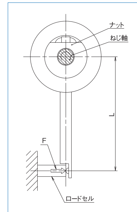
図3 予圧動トルク測定方法
