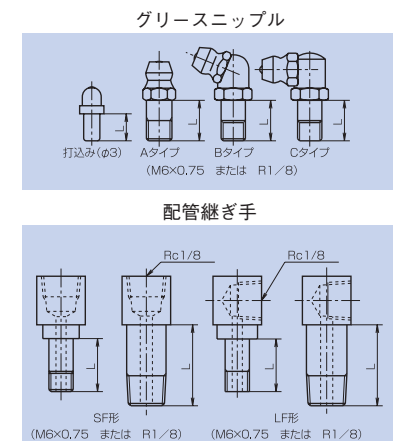
図 3 給油器
