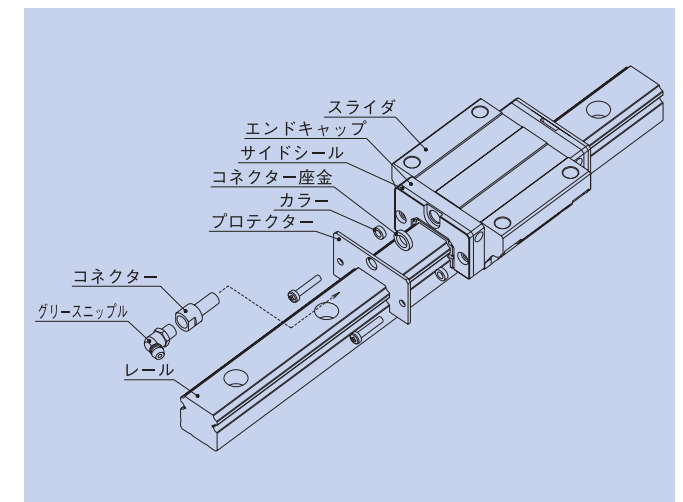
図 17 プロテクター
