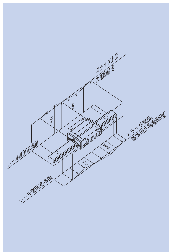
図2 走り平行度
