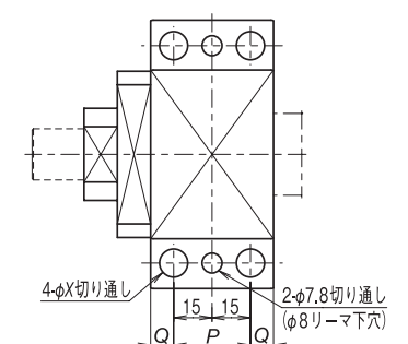
矢視S (WBK25)
