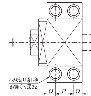
矢視S (WBK17~20)
