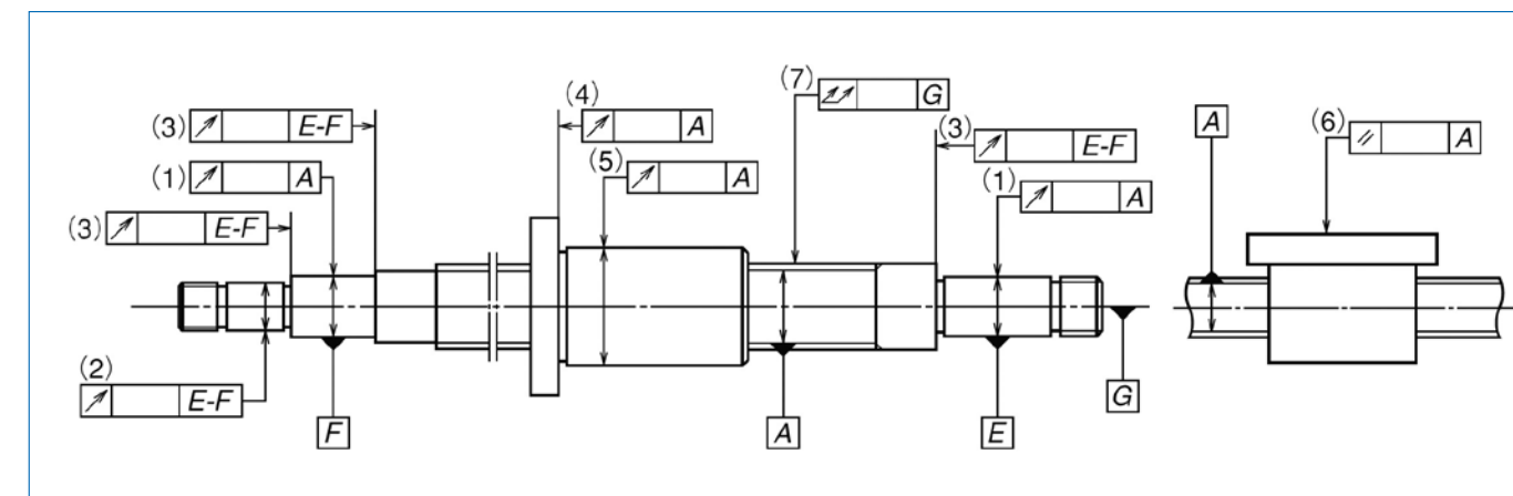
図 2 ボールねじの取付け部精度
