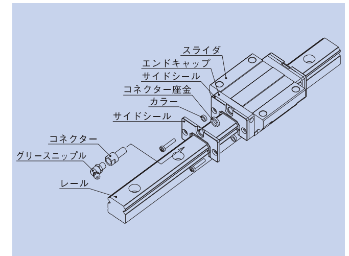
図 16 ダブルシール
