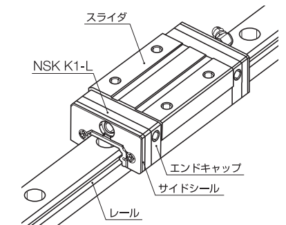
図 2 潤滑ユニット「NSK K1-L™」
