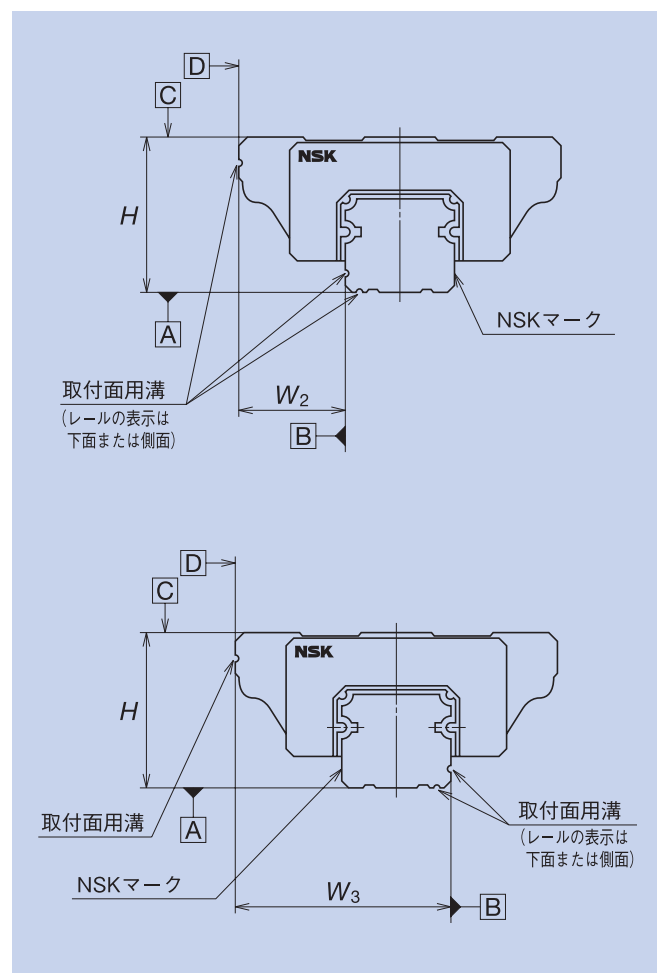
図1 組立寸法
