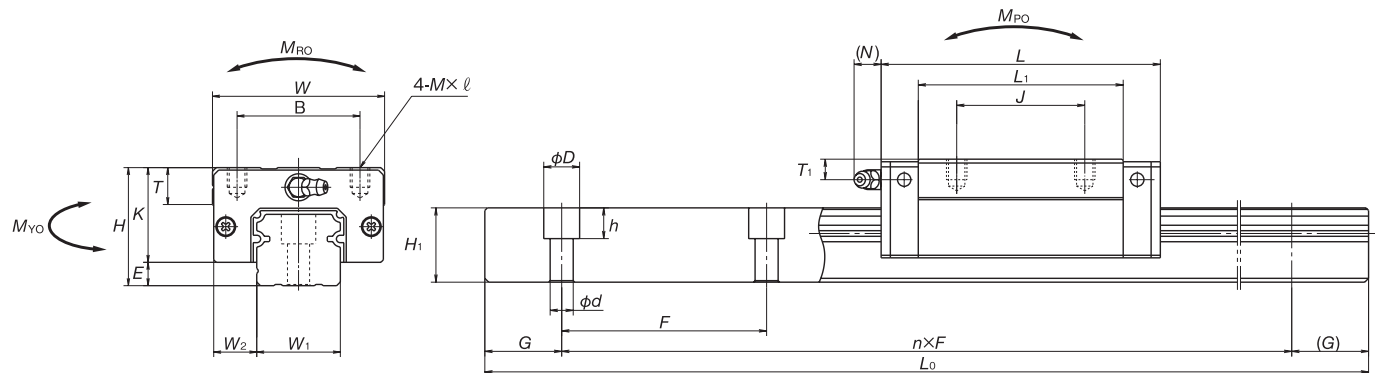
図1 正面図・側面図
