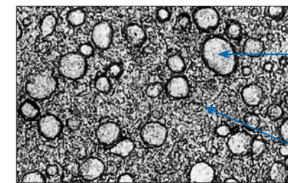
潤滑ユニットNSK K1拡大図 100μm
