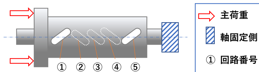
ボールねじ使用例
